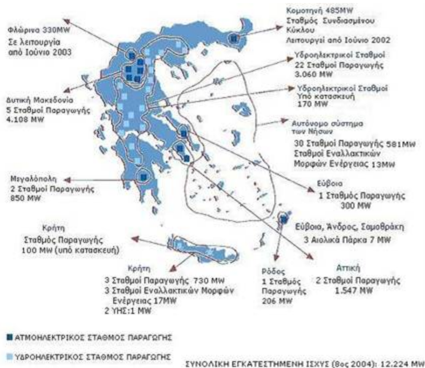
Χάρτης 3: Ατμοηλεκτρικοί και υδροηλεκτρικοί σταθμοί παραγωγής
