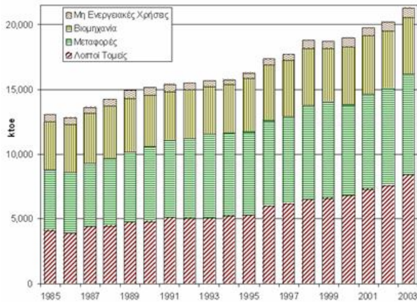
Διάγραμμα 2: Τελική κατανάλωση ενέργειας 1985-2003
