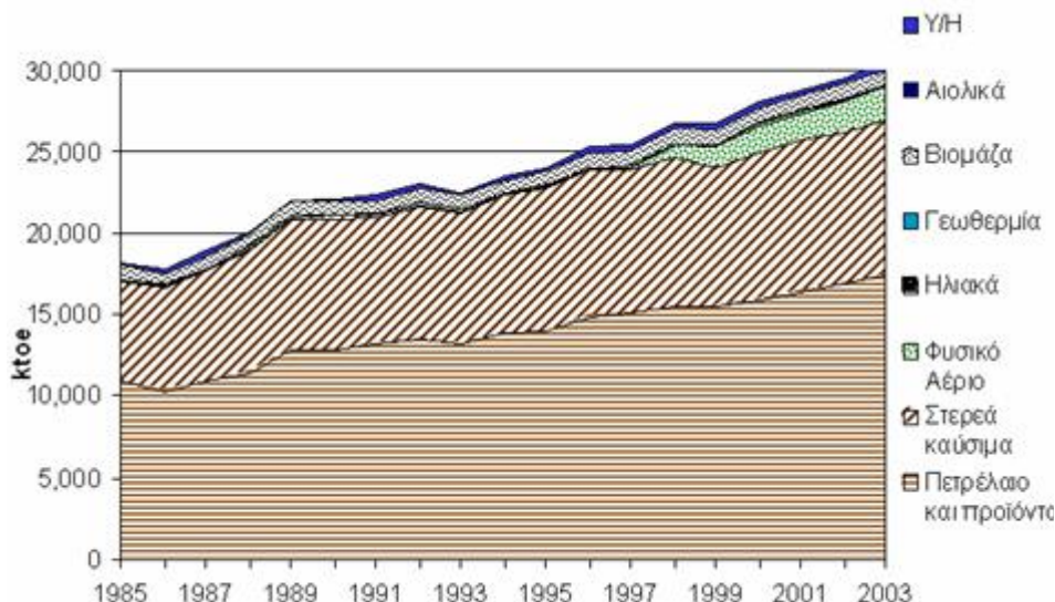
Διάγραμμα 1: Ακαθάριστη εγχώρια κατανάλωση ενέργειας 1985-2003
